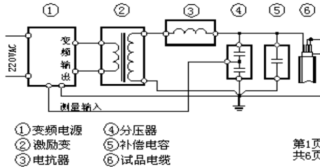
电缆耐压试验接线图A
